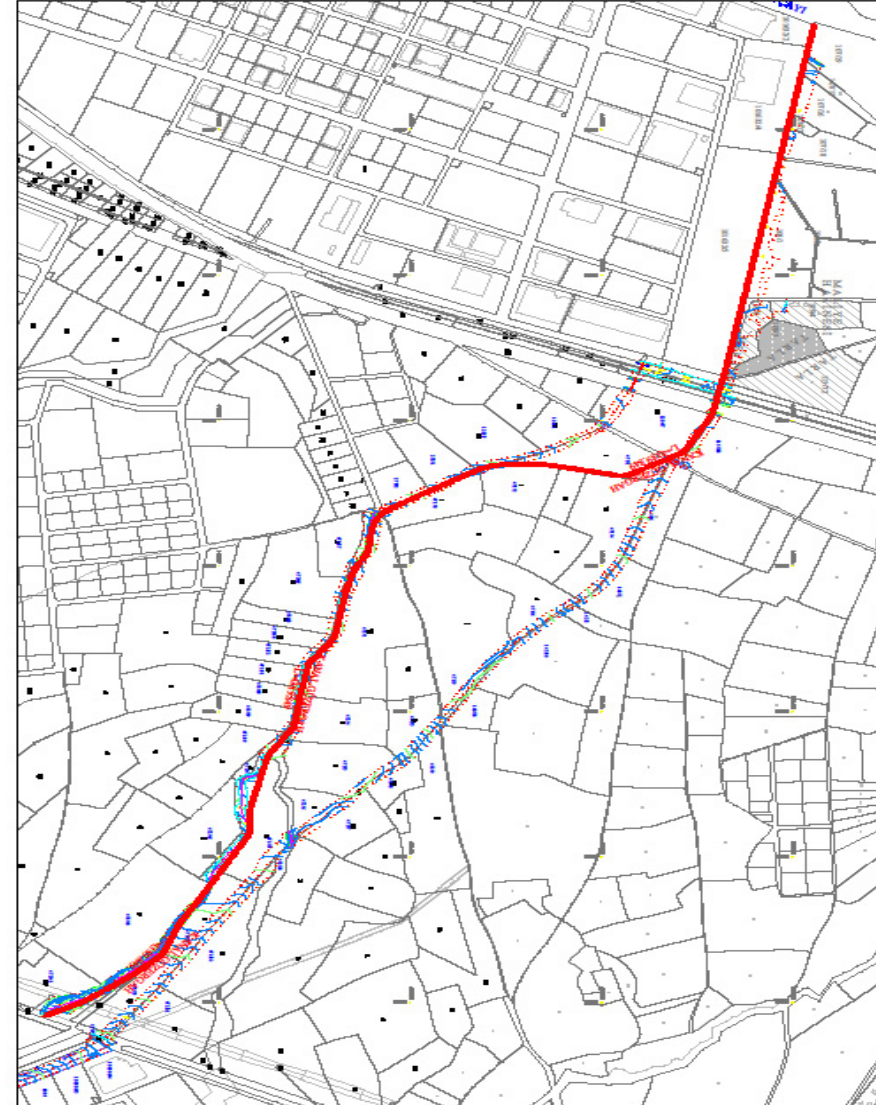
Aritılmış Atıksu Deşarj Hattı Güzergahı
