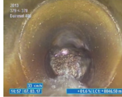
Kanalizasyon hattı iç görüntü
